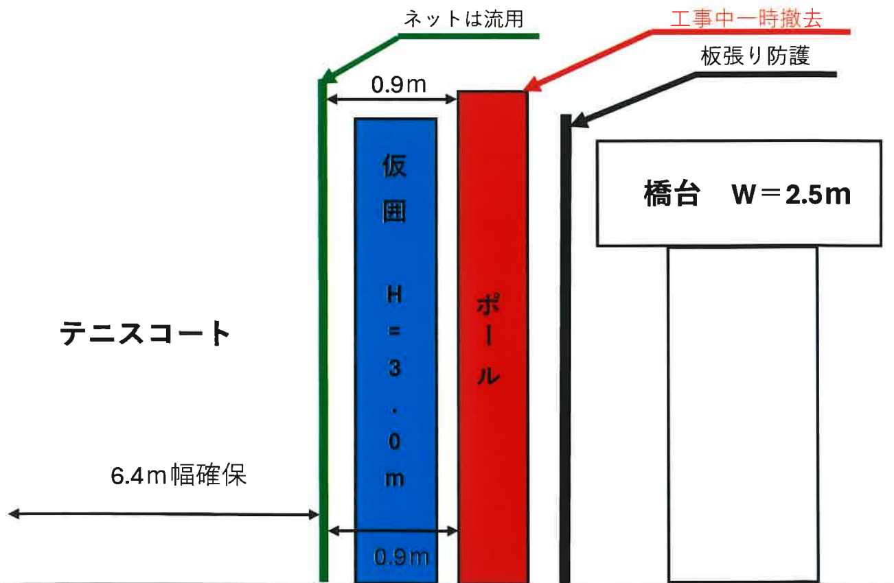
橋台部詳細図
