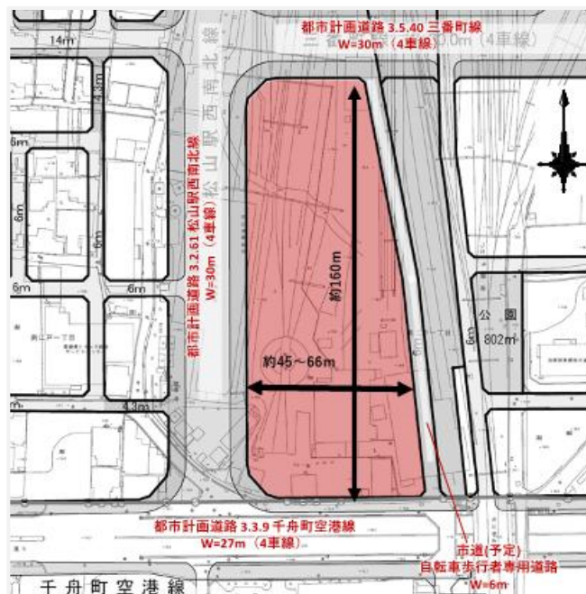
敷地図
