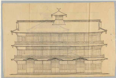
道後温泉本館（神の湯棟）図面 展示施設：振鷲亭
