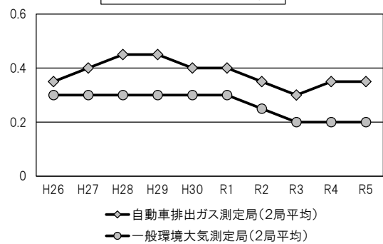
一酸化炭素年平均値の推移
