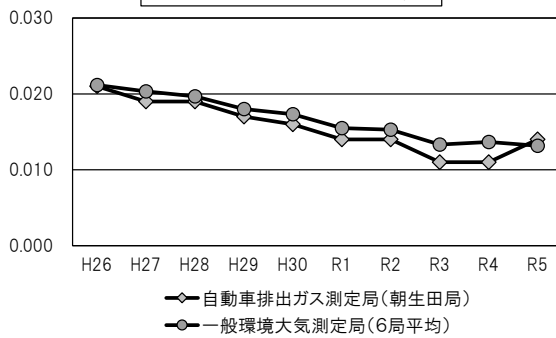
浮遊粒子状物質年平均値の推移
