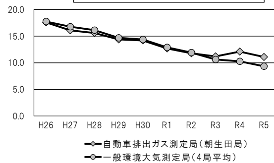
微小粒子状物質(PM2.5)年平均値の推移
