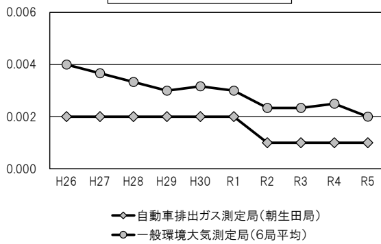
二酸化いおう年平均値の推移
