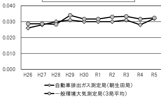
光化学オキシダント年平均値の推移
