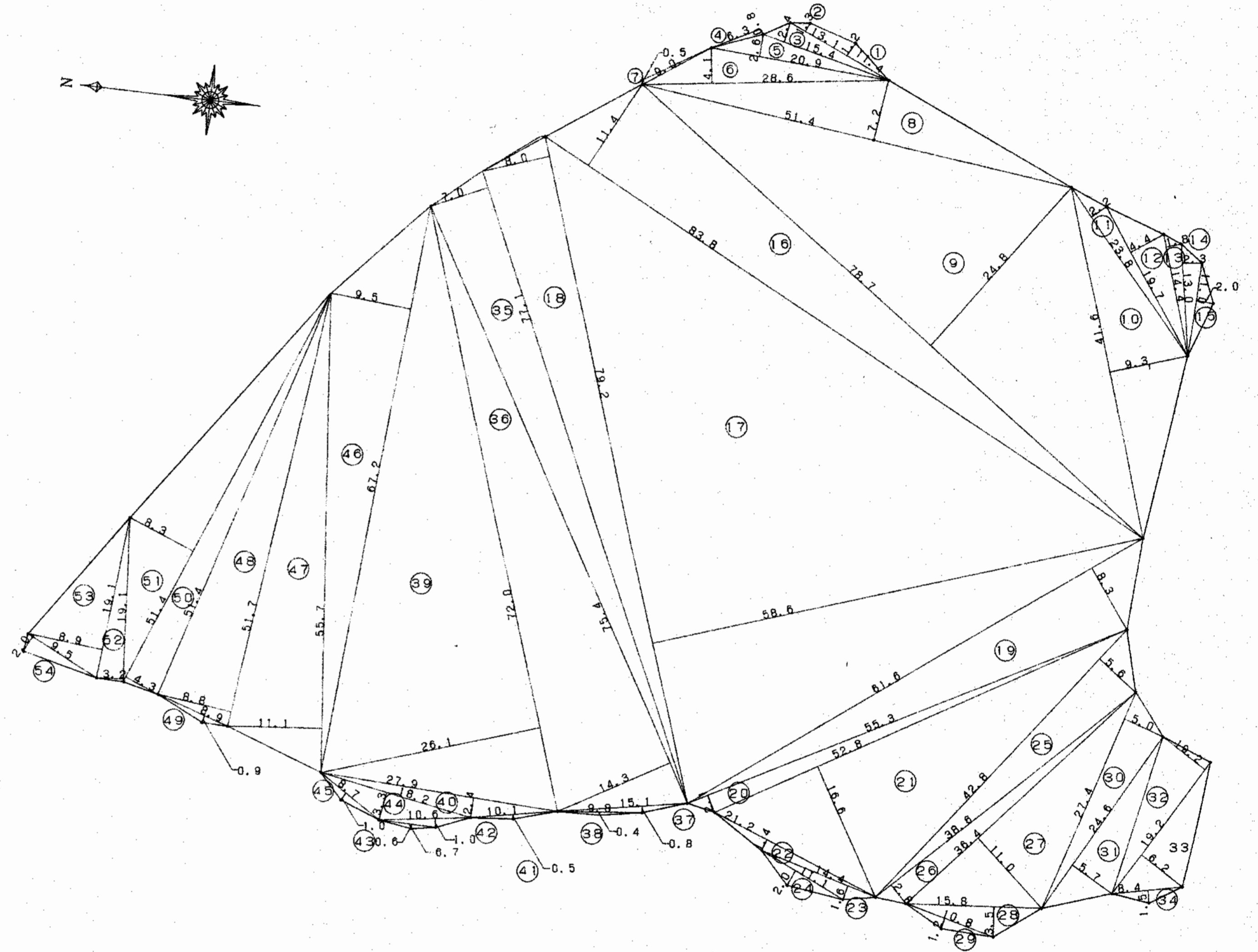
求積図 1/400
