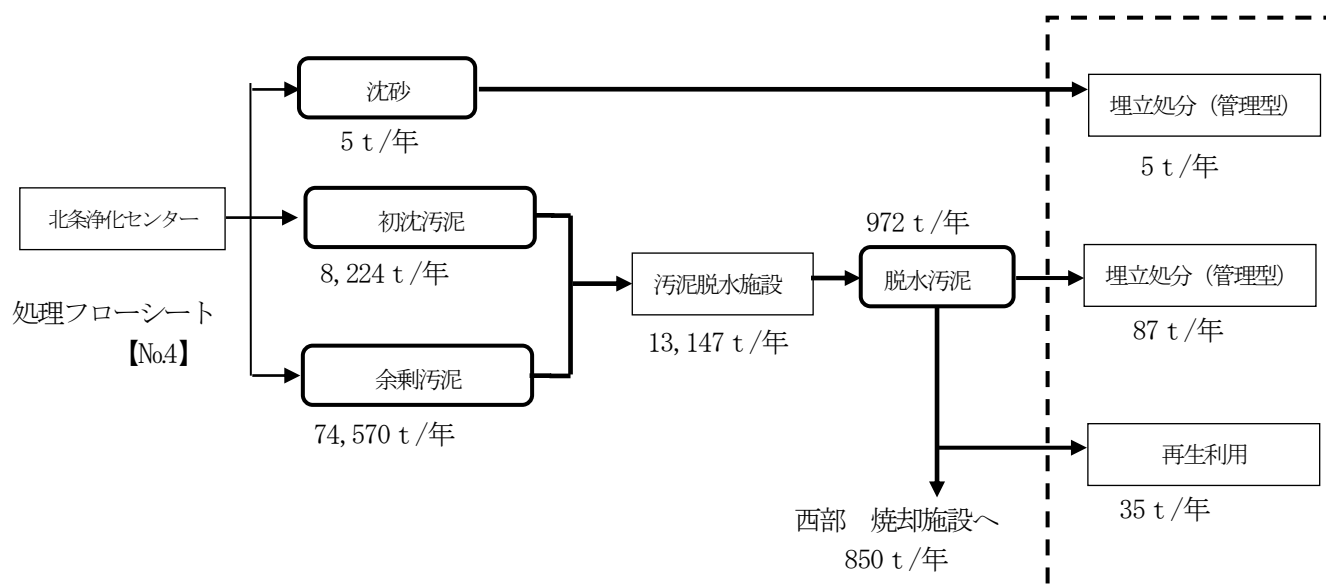
〔図 3-2〕 廃棄物処理フロー図その 2（現状）
