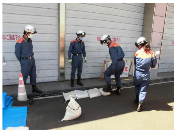
土のう 積み要領
