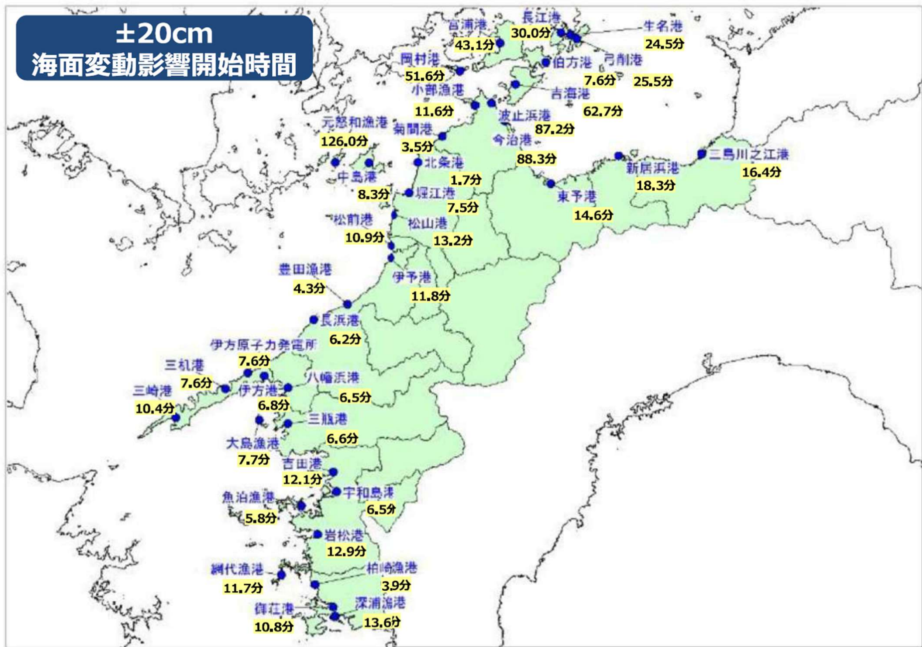
図 3.4-3 海面変動影響開始時間予測図
