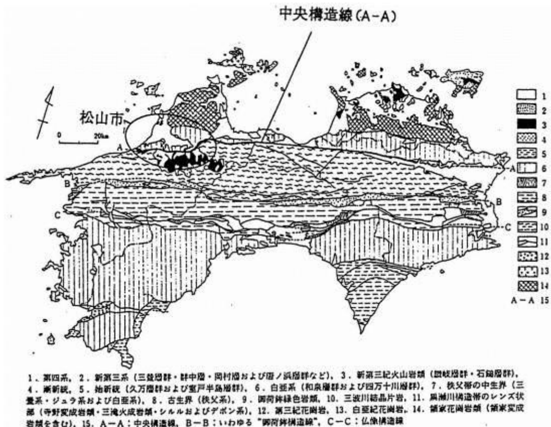
図-1 四国の地質図「基礎I vol114、No.9」
