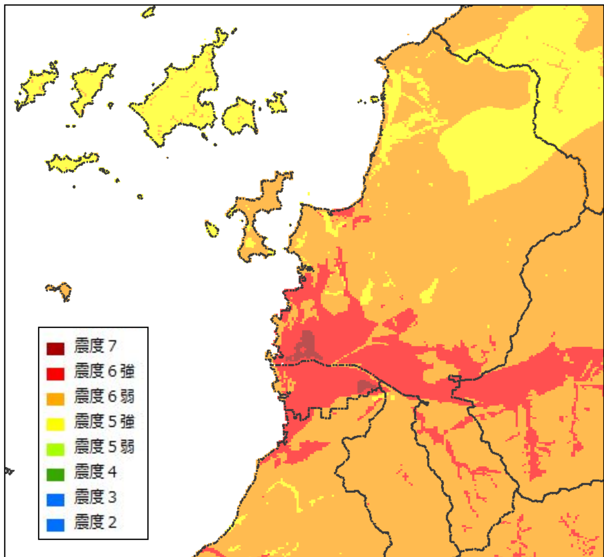
図ー6 推定震度分布図（想定地震Ⅰ：南海トラフ巨大地震（陸側ケース） M9.0） 「愛媛県地震被害想定調査 報告書 平成25年12月」より
