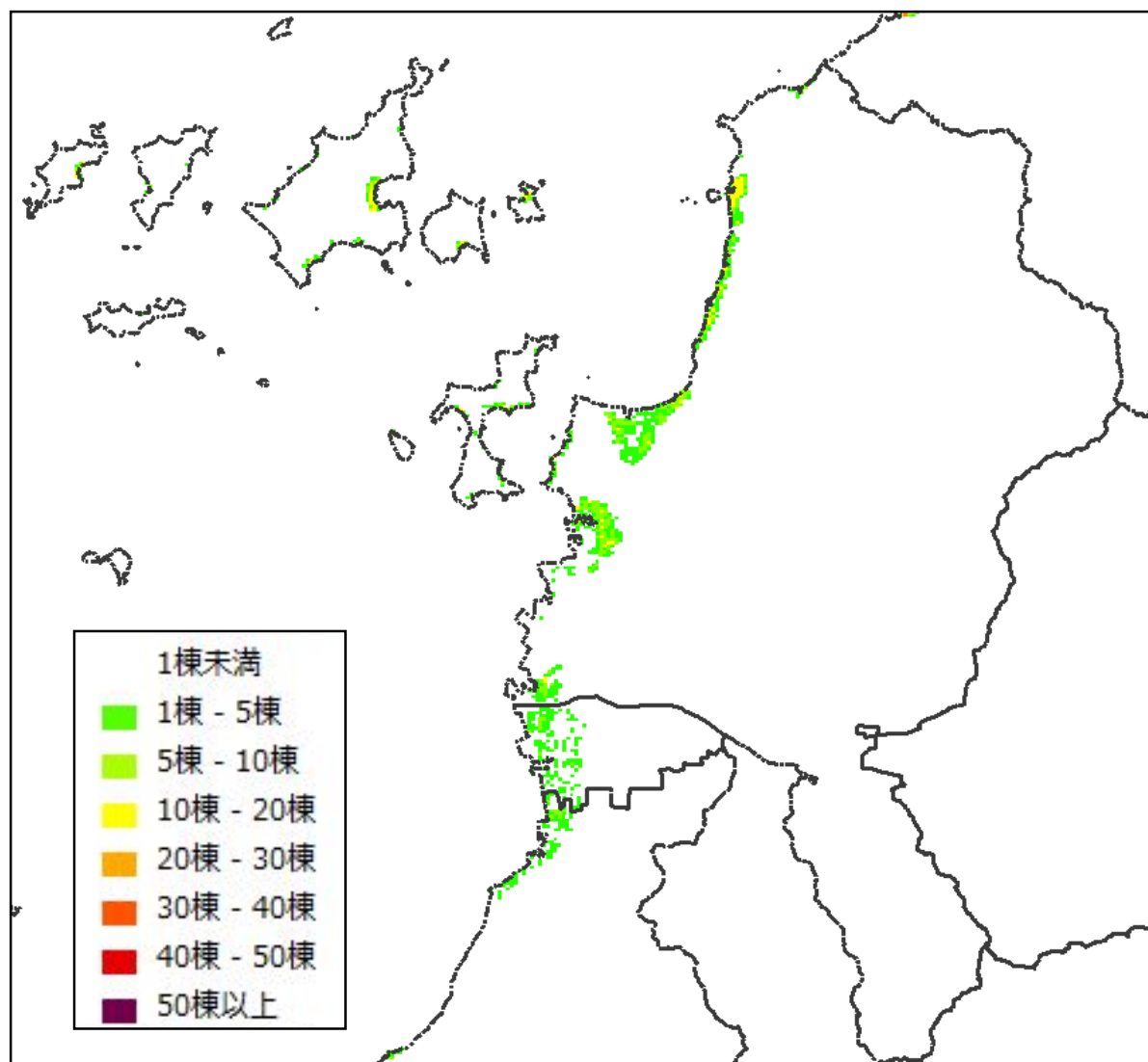
図-13 津波による推定建物半壊棟数分布図 (想定地震Ⅰ：南海トラフ巨大地震（陸側ケース） M9.0) 「愛媛県地震被害想定調査 報告書 平成25年12月」より
