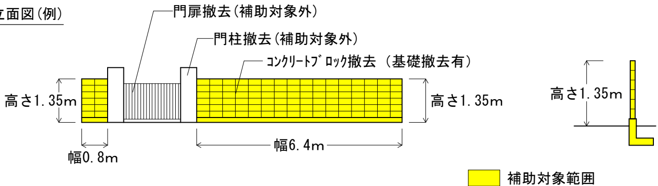
東側立面図(例)
