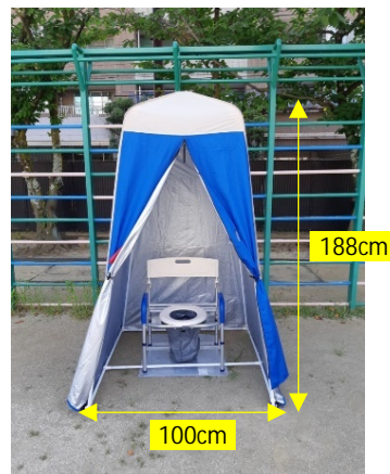
災害用マンホールトイレの便座とテント設置状況
