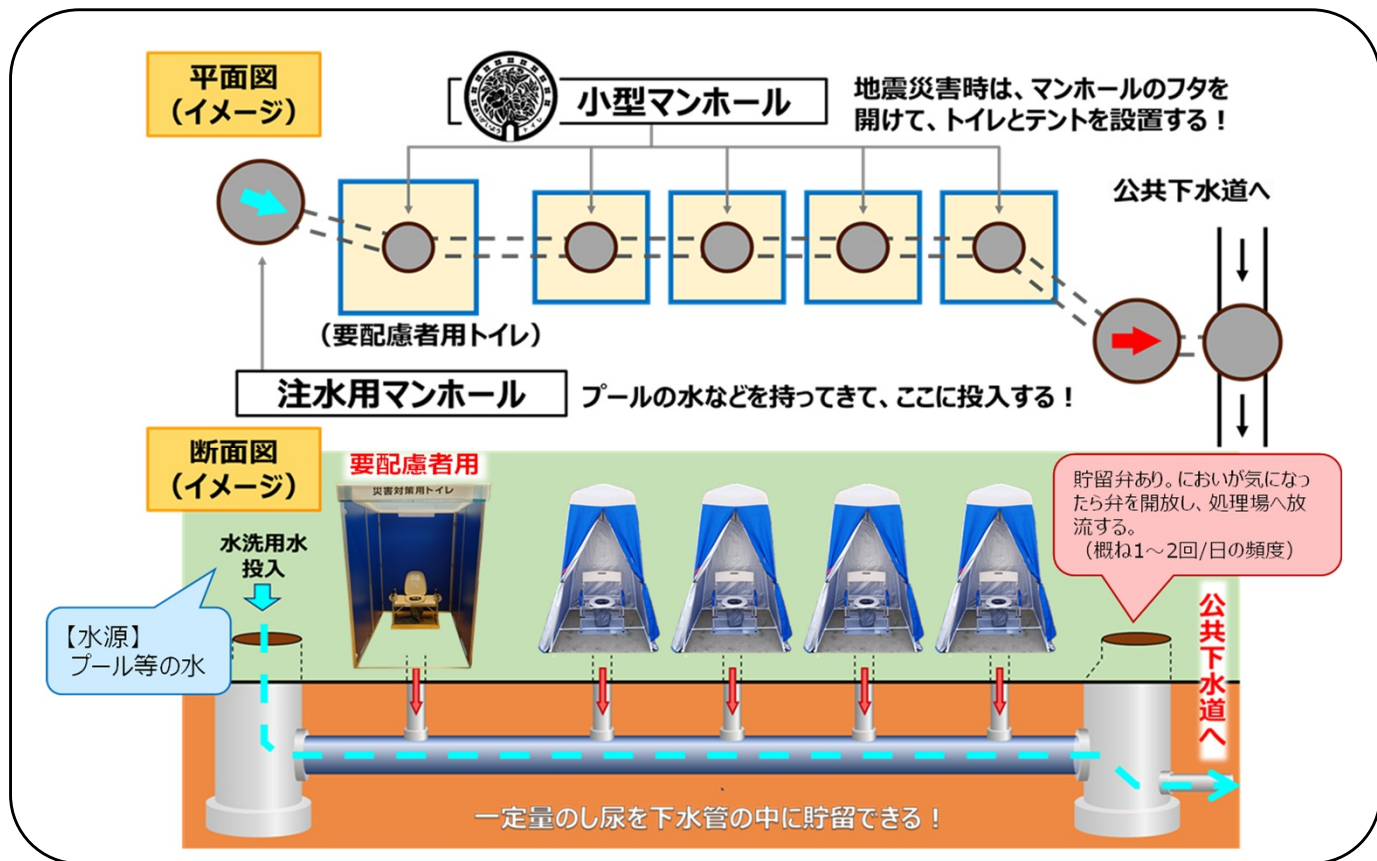
災害用マンホールトイレの仕組み（貯留方式）
