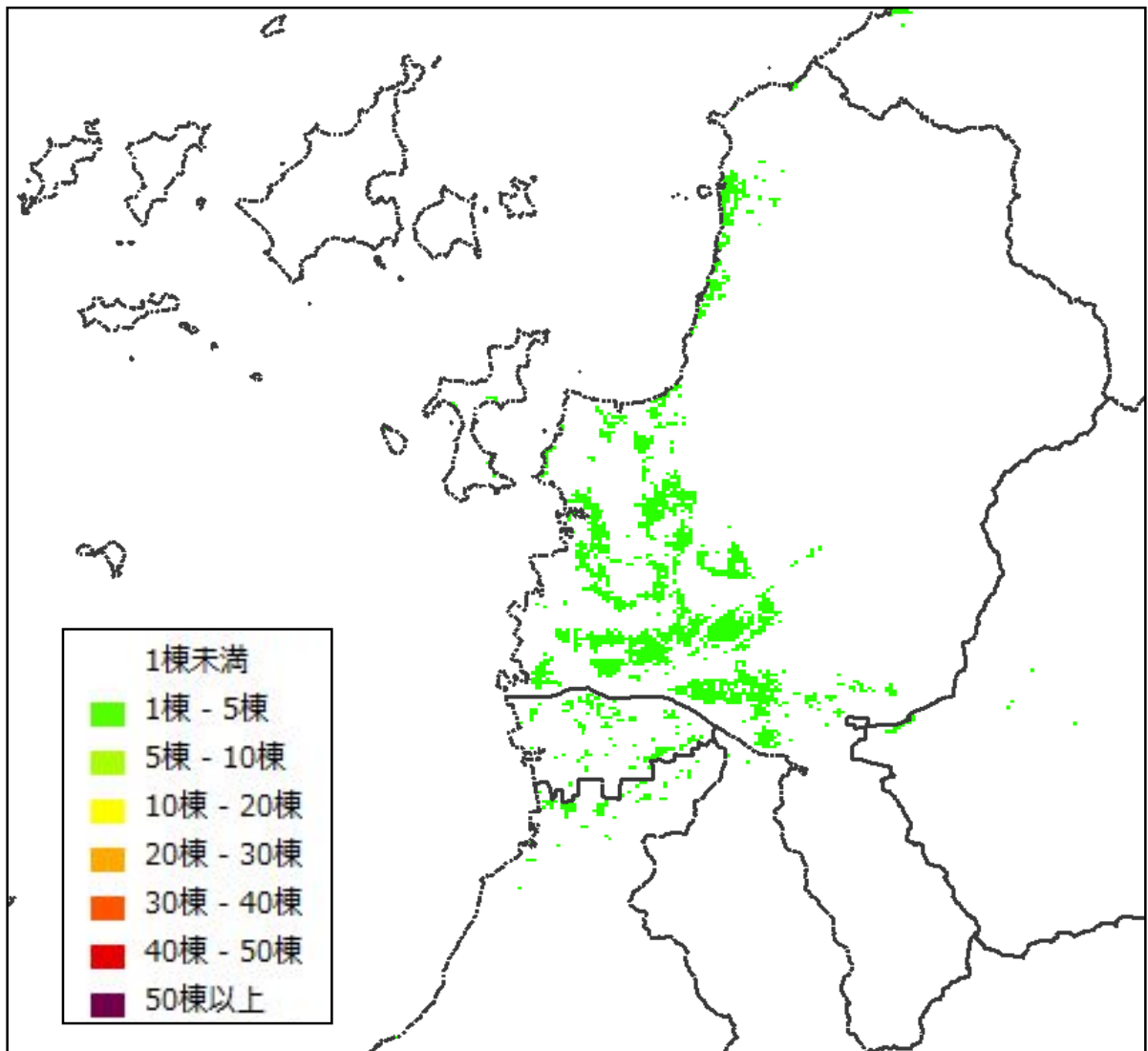
図-11 液状化による推定建物半壊棟数分布図 (想定地震 I : 南海トラフ巨大地震 (陸側ケース) M9.0) 「愛媛県地震被害想定調査 報告書 平成 25 年 12 月」より
