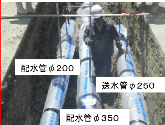
送・配水管の布設状況
