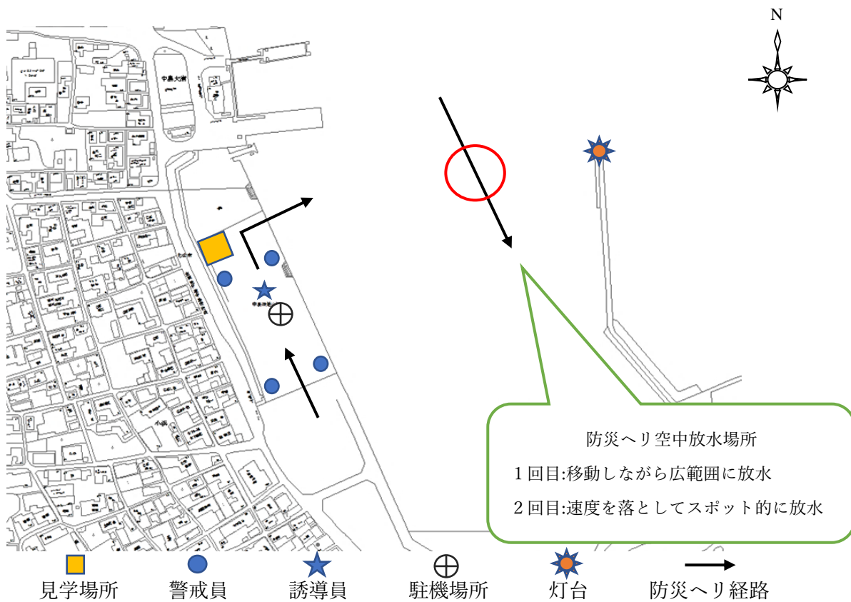
図2 防災へり空中消火放水図
