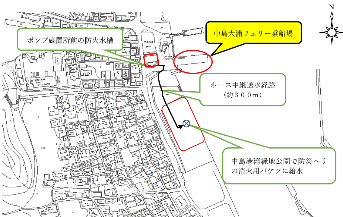
図1 消防団員によるホース中継送水訓練及び消火用バケツ給水訓練図
